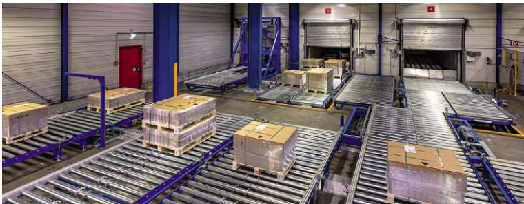
Vertikalförderer-Anlage mit Rollenbahn-Puffer für Paletten
